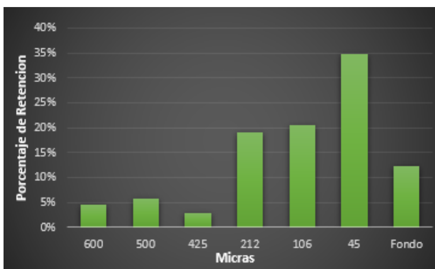
Figura 9. Primer ensayo distribución de tamaño de Partículas de mezcla PET/HPMC.
