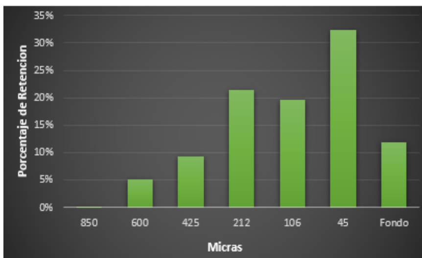
Figura 11. Tercer ensayo de distribución de tamaño de partículas de mezcla PET/HPMC.
