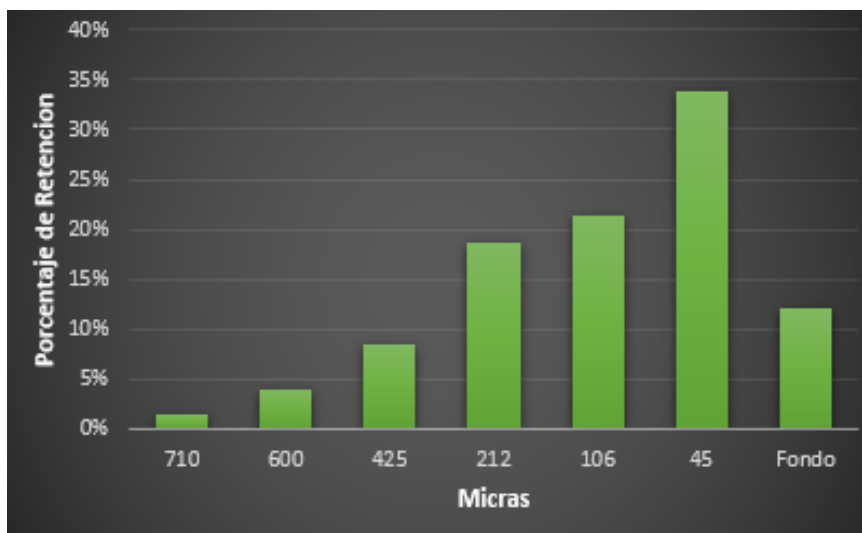
Figura 10. Segundo ensayo de distribución de tamaño de partículas de mezcla PET/HPMC
