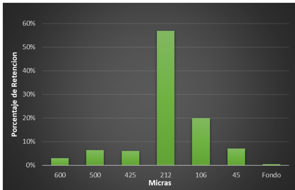
Figura 1. Primer ensayo de distribución de tamaño de partículas del PET
