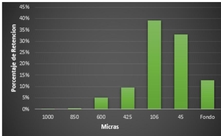
Figura 12. Cuarto ensayo distribución de tamaño de Partículas de mezcla PET/HPMC
